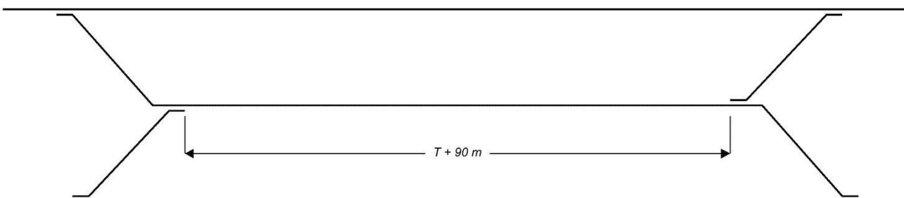
Fig. 5 Flere spor, midtliggende overhalingsspor
