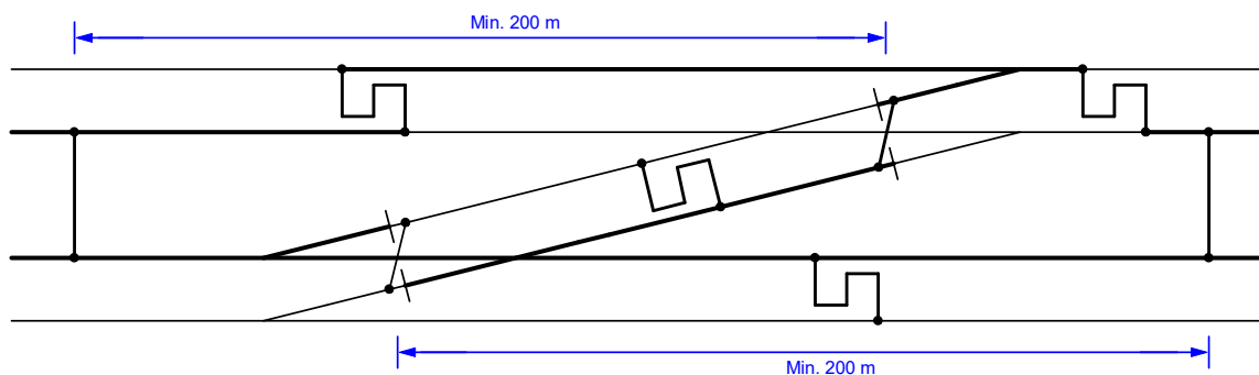
Figur Bilag 4.4-1. Skematisk oversigt over min. afstande på sporforbindere ved sideskift af returskinne på S-banestrækninger med sporløse sporisolationer (FTGS).
