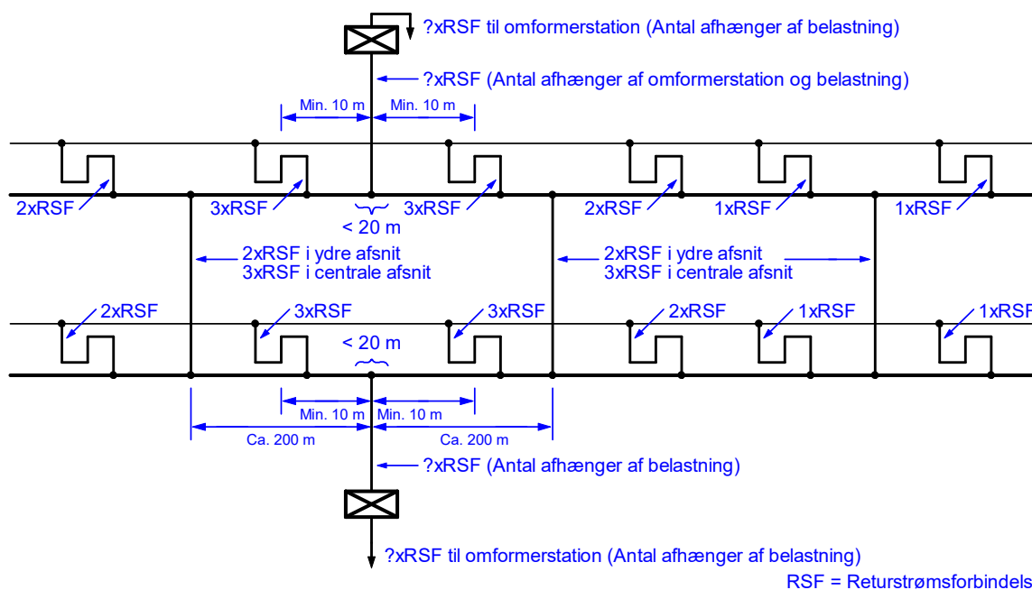
Figur Bilag 4.4-2. Oversigt over tilslutning af returstrømsforbindelser og antal parallelle kabler i returstrømsforbindelser på S-banestrækninger med stødlose sporisolationer (FTGS) i de centrale og ydre afsnit.
