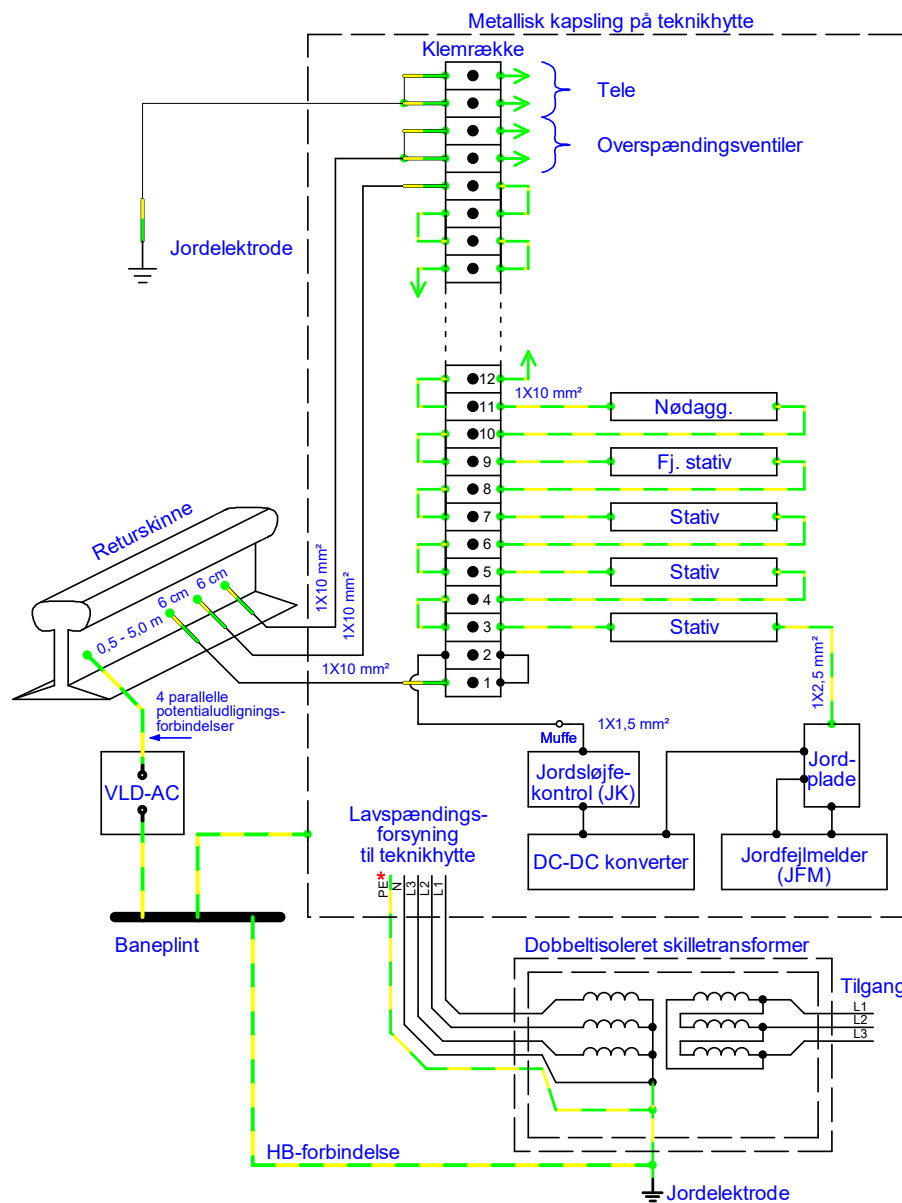
Figur 10.11.1-1. Princip for jording af lavspændingsforsyningen og potentialudligning af udvendige apteringer ved en teknikhytte på en elektrificeret Fjernbanestrækning. Hvis teknikhytten ligger uden for køreledningszonen kan de tre 1X10 mm 2 forbindelser til skinnen i stedet forbindes til en jordelektrode som på S-banen. Det skal beslattes ud fra
