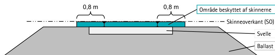
Figur 9.2.6-2. Beskyttelse af apteringer placeret nær skinnerne.
