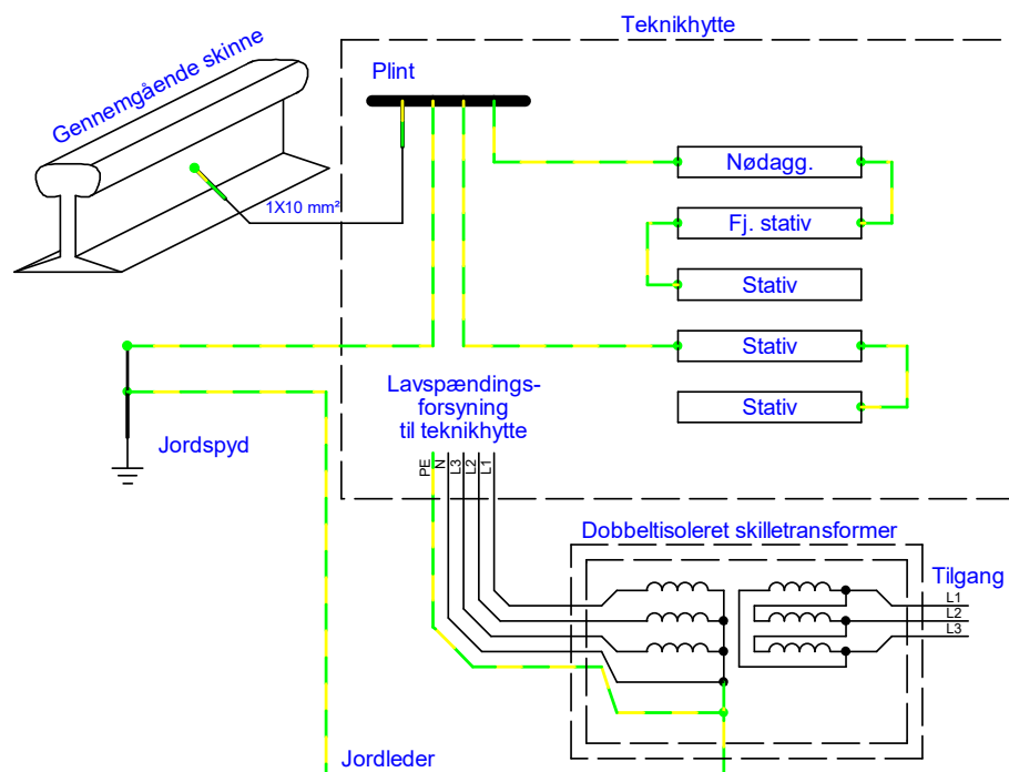
Figur 10.11.1-3. Princip for jording af lavspændingsforsyningen og potentialudligning af udvendige aptringer ved en teknikhytte på en ikke elektrificeret Fjernbanestrækning. Plinten for jording af de indvendige stativer skal forbindes til den gennemgående skinne.
