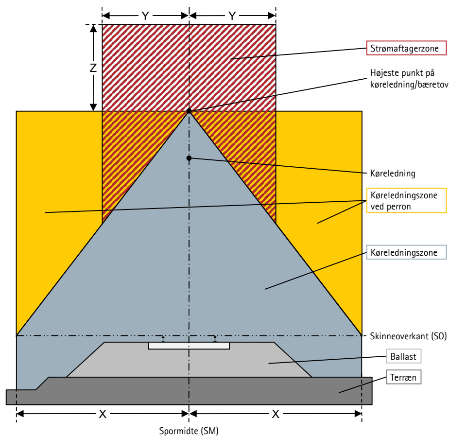
Figur 9.1-1. Profil af køreledningszonen og strømaftagerzonen.
