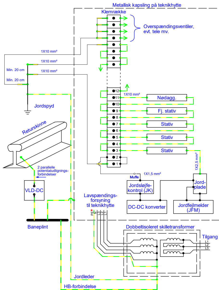
Figur 10.11.1-2. Princip for jording af lavspændingsforsyningen og potentialudligning af udvendige apteringer ved en teknikhytte på S-banen. Sikringsanlægget anvender jordspyd som jordreference. Skitsen er delvist baseret på fig. 2 i SN 299 V nr. 0895 [24].
