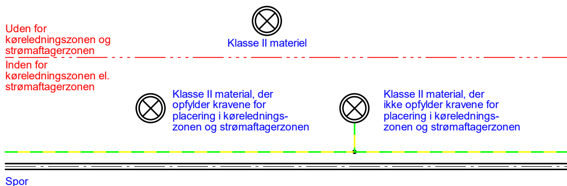
Figur 9.2.5.2-1. Princip for potentialudligning af klasse II materiel.
