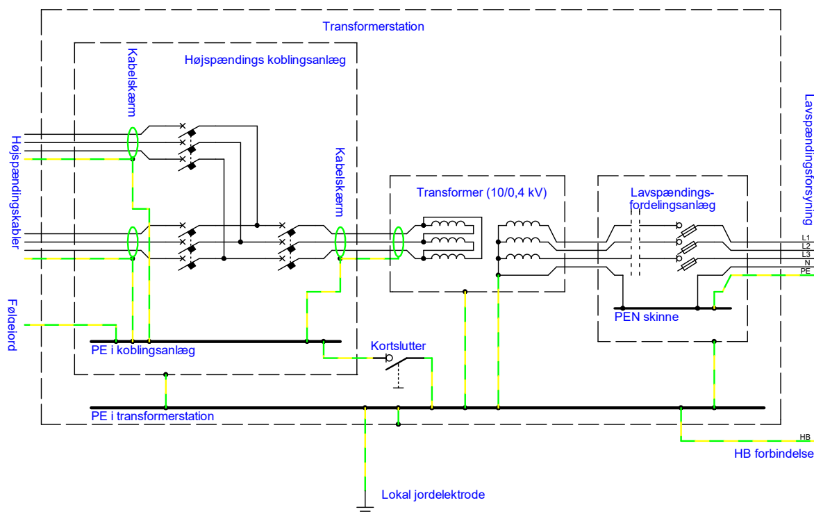
Figur 10.7.2-1. Princip for adskillelse af jordingsanlæg ved anvendelse af TN systemjording med en dedikeret transformestation. Adskillelsen ligger i at jordingsanlægget på højspændingssiden (kabelskærme og følgejord) er isoleret fra det øvrige jordingsanlæg. Der er installeret en kortslutter mellem de to systemer, der kan anvendes ved arbejder i transformestationen. Der kan anvendes TN-C-S eller TN-S (som vist) systemjording fra transformestationen.
