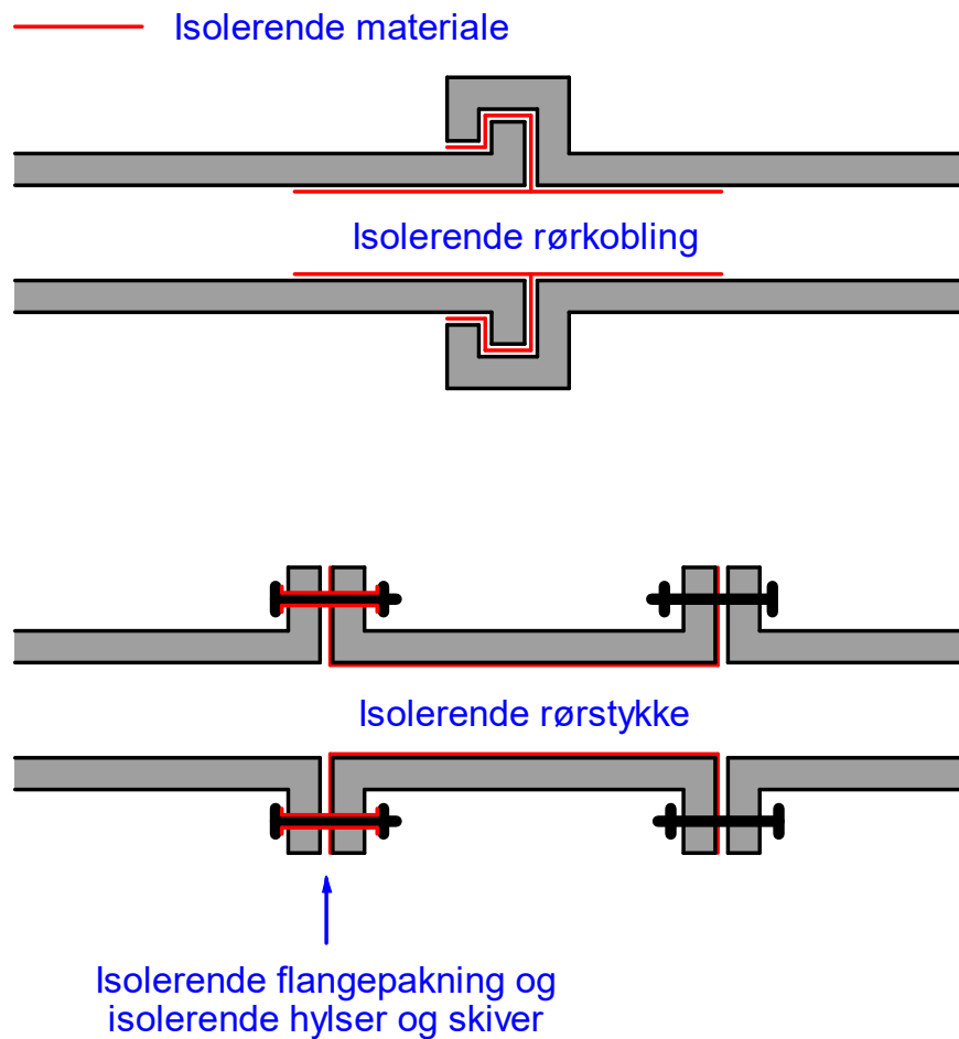
Figur Bilag 6.2-1. Eksempler på elektrisk opdeling i metalliske rør (Illustreret som snit på langs af rør).
