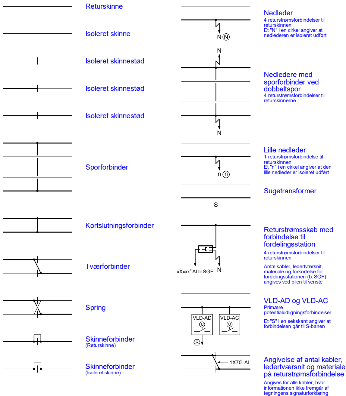
Figur 0-1. Skematisk oversigt over returstrømsforbindelser på Fjernbanen.
