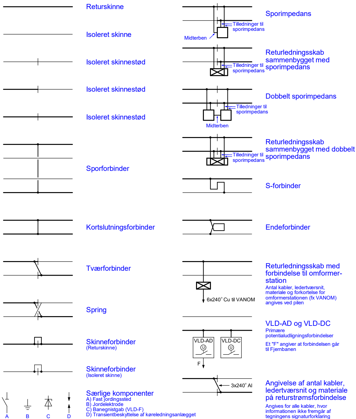
Figur 0-1. Oversigt over returstrømsforbindelser på S-banen.
