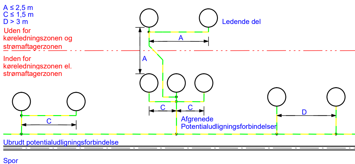
Figur 9.5.5-1. Princip for potentialudligning baseret på ubrudte og afgrenede potentialudligningsforbindelser. Potentialudligningsforbindelsen parallelt med sporet er en ubrudt potentialudligningsforbindelse, mens alle de øvrige er afgrenede potentialudligningsforbindelser.
