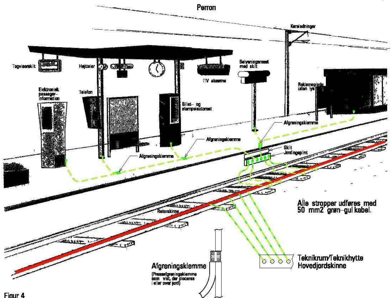
Figur 4 Fjernbanen Eksempel på beskyttelsesjording på station
