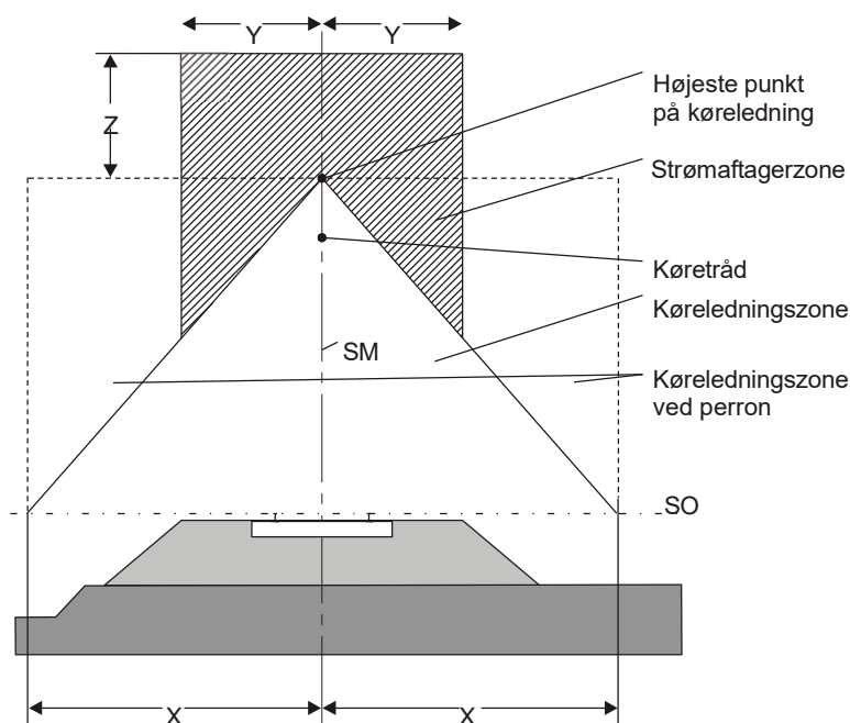
Figur 11.1-1: Køreledningszone og strømaftagerzone.
