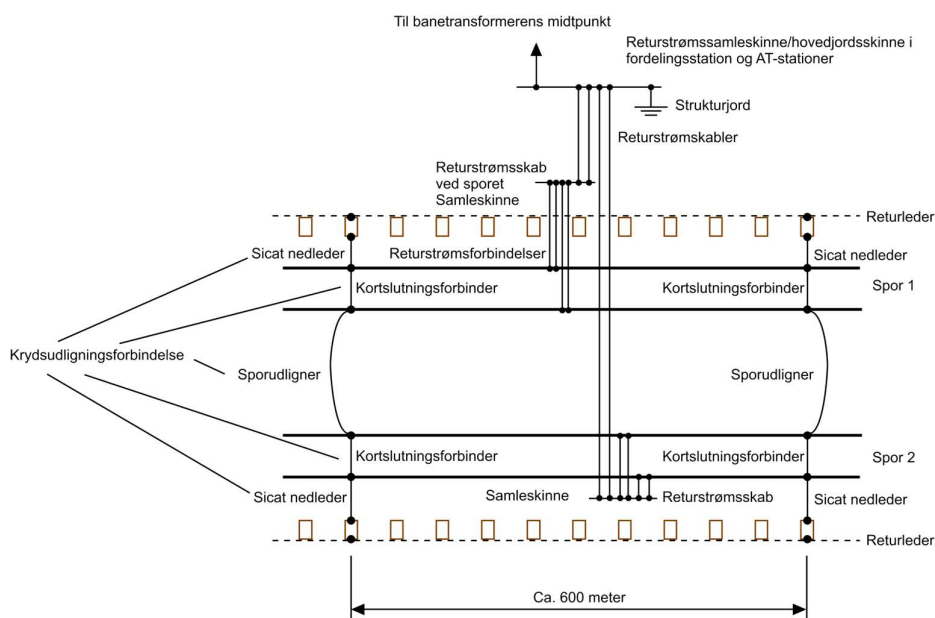
Figur Bilag 8.1-1 Principdiagram for returstrømsforbindelses-/kabernes tilslutningspunkter for et dobbeltspor.
