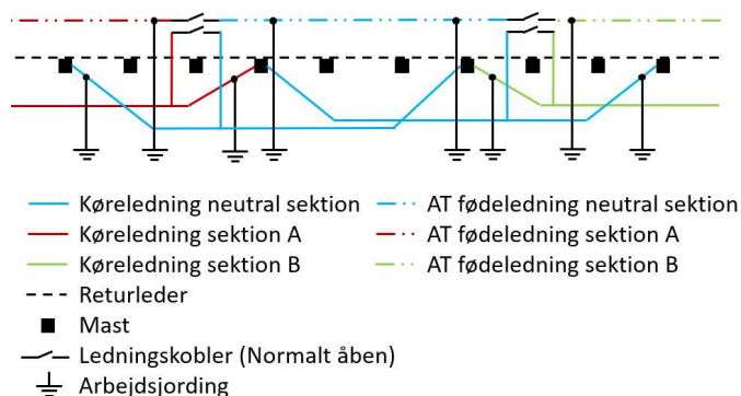
Figur 11.8.1-2 Arbejdsjording i "split" neutralsektion.
