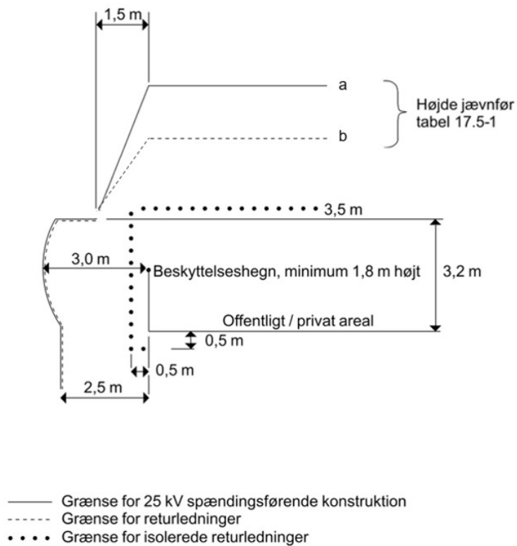
Figur 17.5-2 Grænser for placering af køreledningsanlæg nær offentlige/private arealer (veje, stier, pladser og lign.) med beskyttelseshegn i skel.
